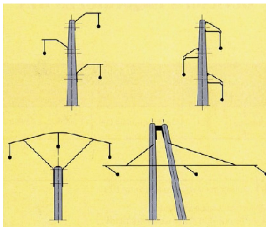
Figure 4 : Réseau électrique HTA nu - Technique suspendue
