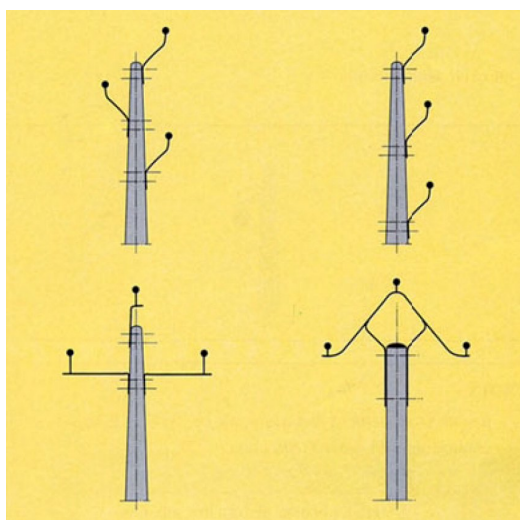
Figure 3 : Réseau électrique HTA - Technique rigide
